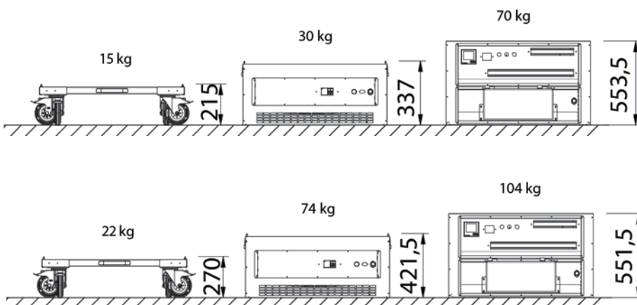
Abb.1 Wärtsilä JOVYLOAD EASY und EASY XL in 3 Teile zerlegt
